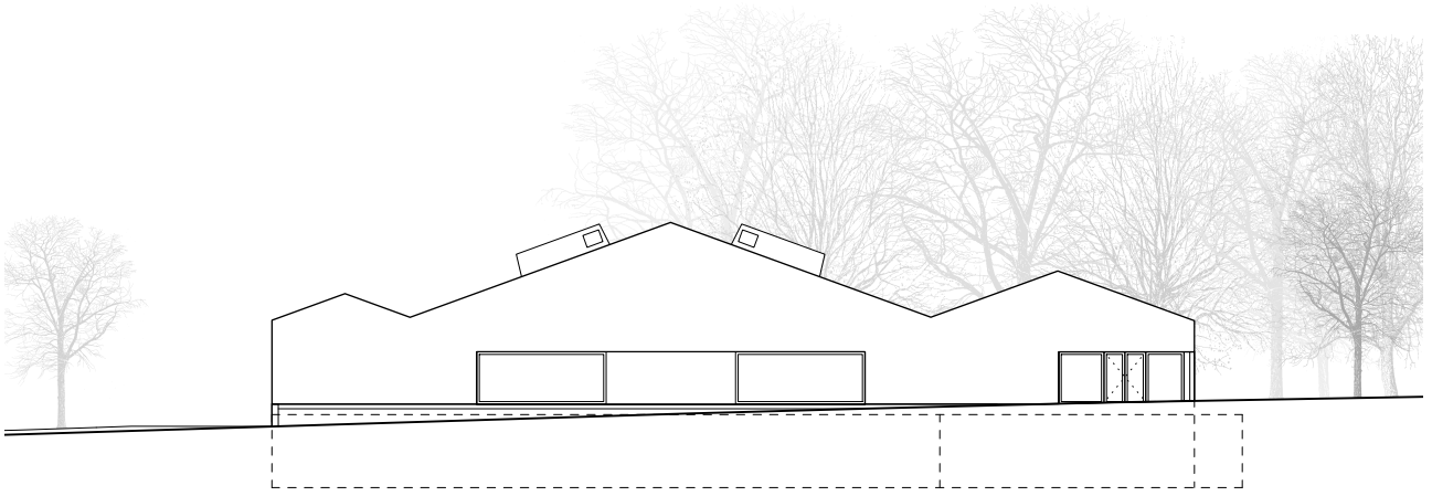
Nordfassade
